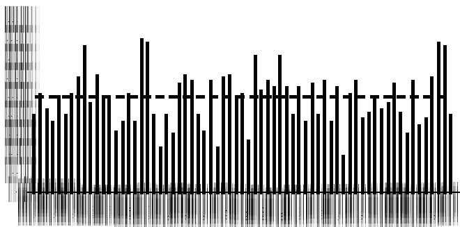
Figure 1 : Pluviométrie totale annuelle à l'aéroport de Marrakech pour la période 1932-1998. La Pluviométrie moyenne est indiquée en pointillé.
